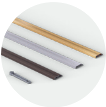
Metalen Incizo-profiel QSINCPR(-) 2.700 x 47 x 11 mm
